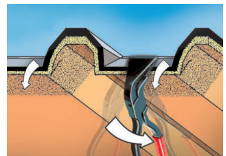
Profilblech mit einer angesetzten Falzzange ca.1,5 cm nach unten anbiegen
