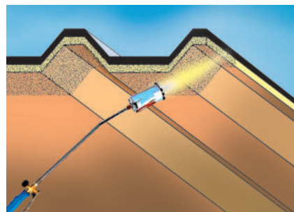
Schmelzen mit Gasbrenner (alternativ)
