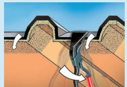
Profilblech mit einer angesetzten Falzzange ca.1,5 cm nach unten anbiegen
