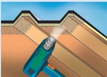
Schmelzen mit Heißluftpistole (ca. 650.)
